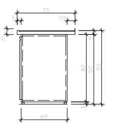
Schnitt C-C
